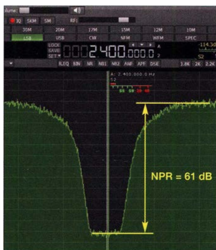
Bild 13: Bei einem Tiefpassfilter am Antenneneingang verbessert sich das NPR.
