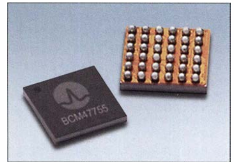
Bild 3: Broadcom BCM4775 – Satellitenempfänger-IC der 3. Generation Werkfoto
