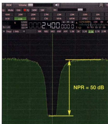
Bild 12: Messung des Rausch-Leistungs-Verhältnisses am Empfänger Colibri-Nano
