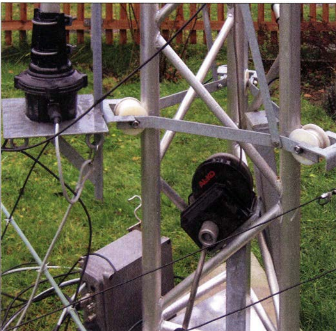
Bild 11: Das Foto zeigt die untere Seite des Schlittens, die den Mast umfassenden Gleiter mit den Rollen, die aus T-Material gefertigten Verbindungsstreben zwischen oberem und unterem Gleiter sowie die stabilisierende Querstrebe aus Flachstahl. Man sieht den Windenbock im Mast, die Rotorplattform, die Einhängösen für Kabel etc. Am Boden liegt der Antennenumschaltkasten, der nach Hochfahren des Schlittens wieder in den Mast eingehängt wird.
