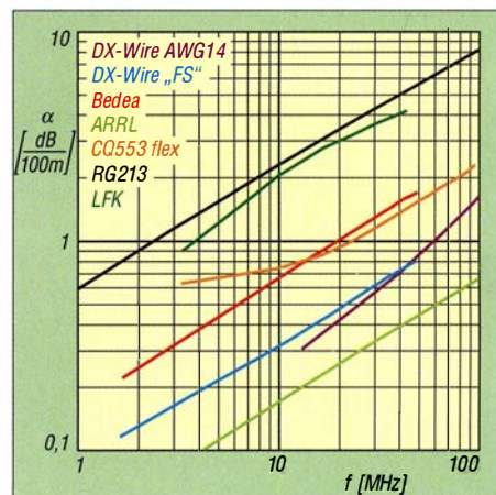
Bild 2: Dämpfungskonstante \alpha unterschiedlicher Koaxialkabel und Zweidrahtleitungen im Vergleich
