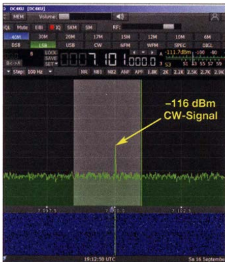
Bild 9: Signal-Rausch-Abstand von 3 dB bei einem HF-Signalpegel P = -116 dBm
