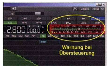
Bild 8: Bei zu hohem Rauschpegel erfolgt eine Übersteuerung des SDR.
