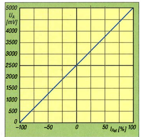
Bild 8: Der MLX91208 liefert ein zur Stromstärke lineares Ausgangssignal.
