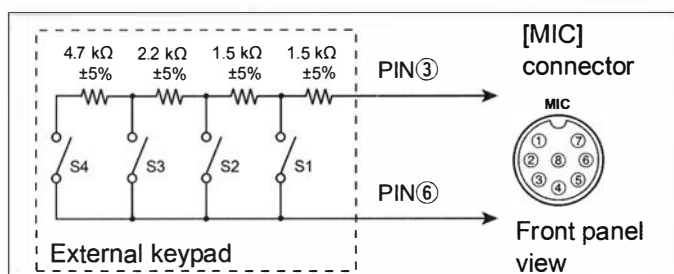
Bild 3: Originalschaltplan gemäß Handbuch für das externe Zusatzgerät zum Abruf der ersten vier Speicherplätze beim IC-7300
