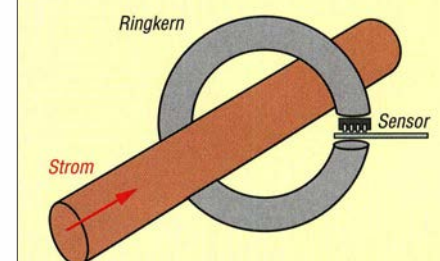
Bild 4: Bei der Messung geringer Stromstärken ist das Magnetfeld des Leiters durch einen Weicheisenkern zu bündeln.
