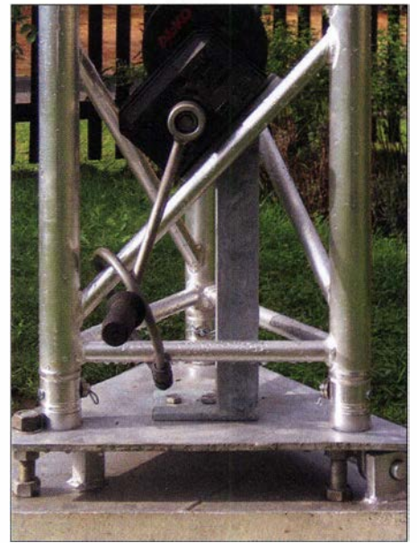
Bild 12: Unterkonstruktion mit Winde und Fixierung mit einem Fahrradschloss
