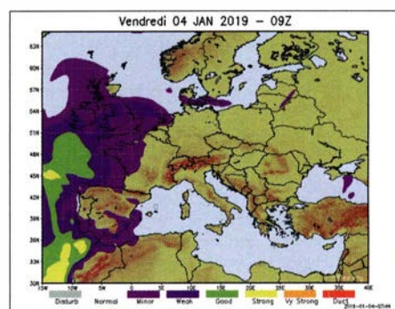
Die aus dem Hoch resultierenden Überreichweiten wurden abermals auf der F5LEN-Karte nur als „minor“ bis „weak“ klassifiziert. Man mag sich gar nicht vorstellen, was in den als „good“ oder „strong“ bezeichneten Zonen los sein könnte. Grafik: F5LEN
