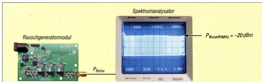
Bild 1: Das konstante Signalspektrum des Rauschgenerators reicht von nahe 0 Hz bis in den Gigahertzbereich (hier bis 200 MHz auf dem Bildschirm des Spektrumanalysators).
