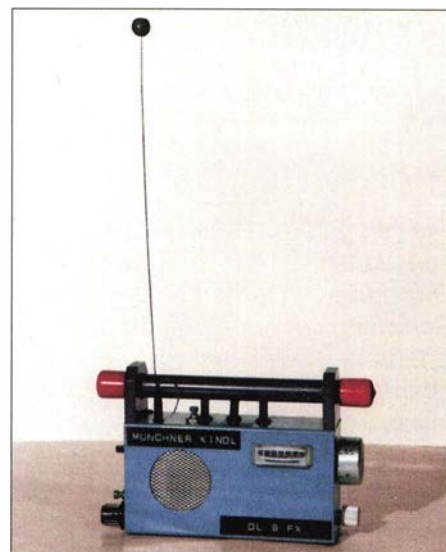
Original des 80-m-Peilempfängers „Münchner Kindl“ von Günter Hoffschildt, DL9FX; Bauanleitung erschienen in CQDL 3/1975
