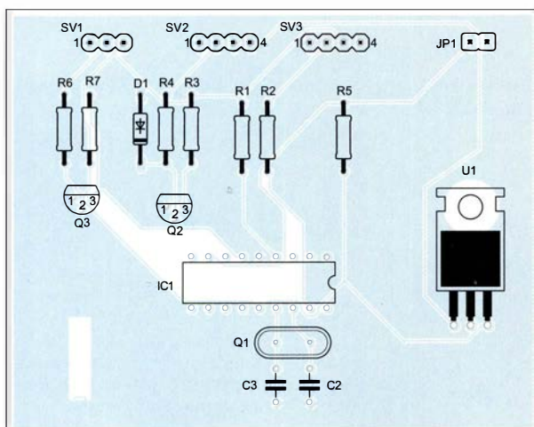
Bild 5: Bestückungsplan der einseitig kupferkaschierten Leiterplatte für die Steuerung mit einem PIC; Abmessungen 63 mm × 80 mm, M 1:1; der Aufbau ist gleichfalls auf einer Universalleiterplatte möglich.
