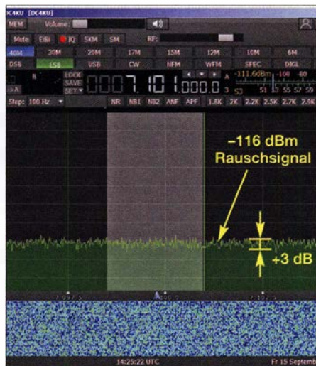
Bild 10: Rauschanstieg um 3 dB bei einem eingesperrten Rauschpegel P_{\text{Noise}} = -116 dBm
