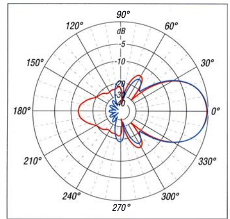
Bild 6: Unter Freiraumbedingungen simulierte Elevationsdiagramme der OK1DE- (rot) und der neu entwickelten DK7ZB-Yagi (blau); äußerer Ring 0 dB ± 11,35 dBd
