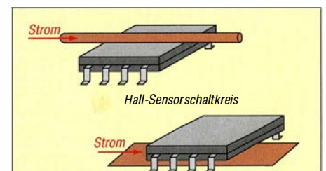
Bild 3: Zur Strommessung ist eine Leitung über dem Hall-Sensor oder eine Kupferfläche darunter anzuordnen.
