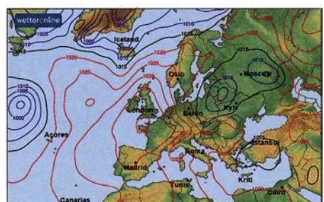
Dieses kräftige Hoch mit Kerndruck 1040 hPa sorgte Anfang Januar für tagelange troposphärische Überreichweiten auf 144 MHz und höheren Bändern. Grafik: www.wetteronline.de
