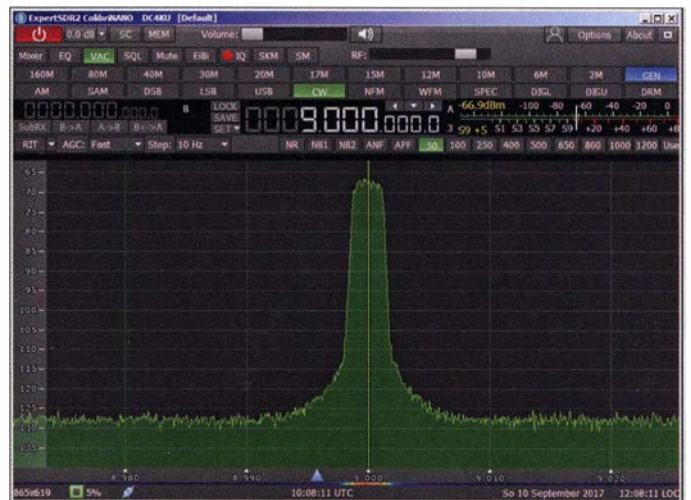
Bild 5: Übertragungskurve eines Roofing-Filters mit 12 kHz Bandbreite
